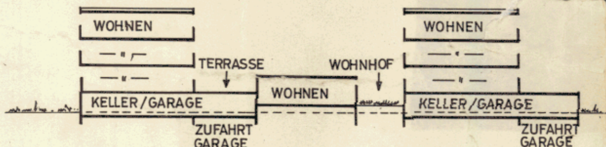
SCHNITT A-B M 1:400
